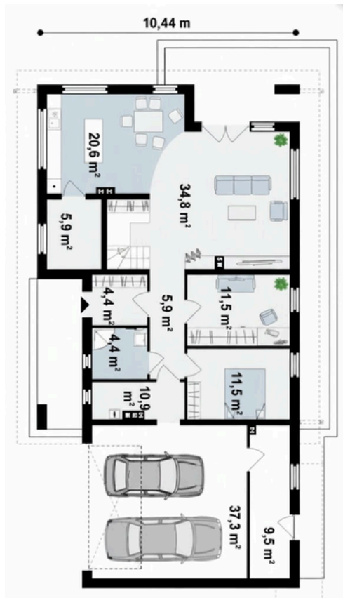
Planta Baja
